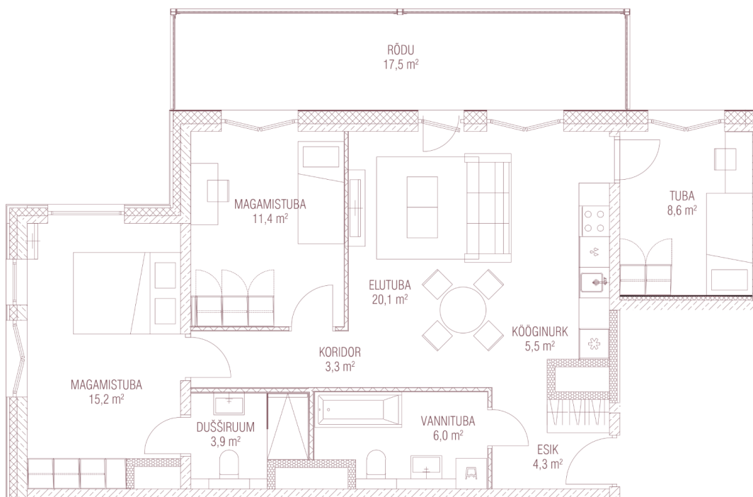
Taludevahe 57
